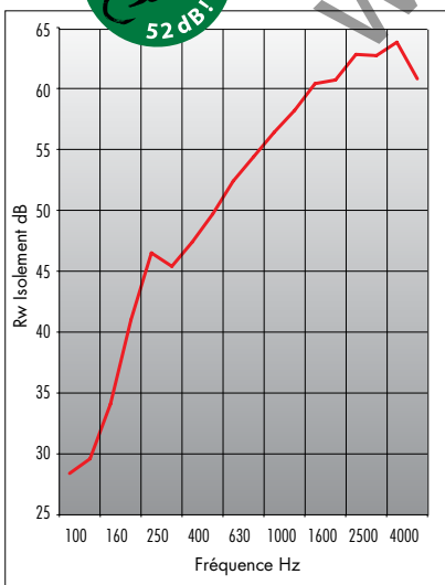
Extension essai CEDIA 06/4861 Sous-toiture Fibro-plâtre sur profil
